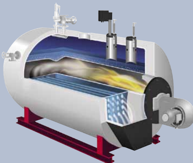
Eclaté d'une chaudière moderne trois parcours avec un volume d'eau relativement faible.
